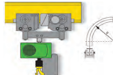
Siirtovaunu pienellä kääntösäteellä
