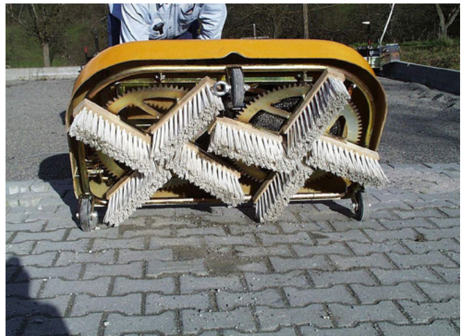
Levittimen harjat
