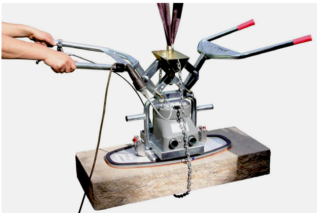
SPEEDY VS-140/200
