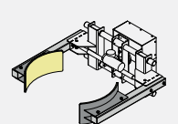
Tynnyrinkääntölaite 87925 Gripper D
