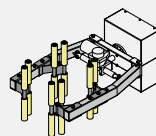
Tynnyrinkääntölaite 87924 Gripper B
